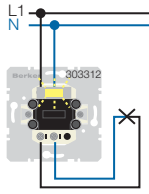
Ausschaltung 2-polig Dauerbeleuchtet (Glimmaggregat 160002 leuchtet immer)
