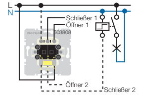
Wippentaster mit getrennten Eingangsklemmen (2 Wechsler). Glimmaggregat 160002 leuchtet wenn Stromstoßschalter aus
