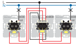
Wechselschaltungen mit Doppelwechschalter inklusive Glimmaggregat 160002 (auch unbeleuchtet möglich) (Glimmaggregat am Doppelwechschalter leuchtet nur wenn rechte Schaltung aus)
