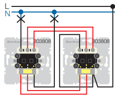
Doppel-Wechselschaltung beleuchtet mit Glimmaggregat 160002 (Leuchtet nur wenn linke Schaltung aus)
