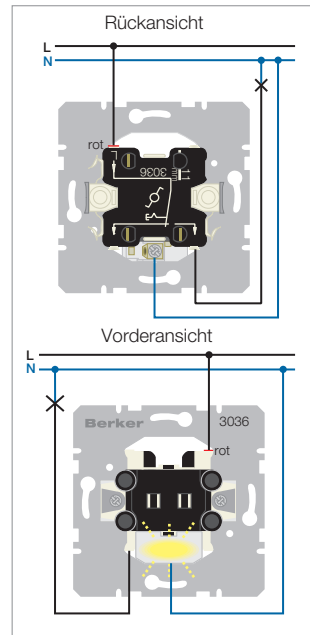
Ausschaltung Kontrolle mit Wechselschalter (Glimmaggregat leuchtet bei "Ein")
