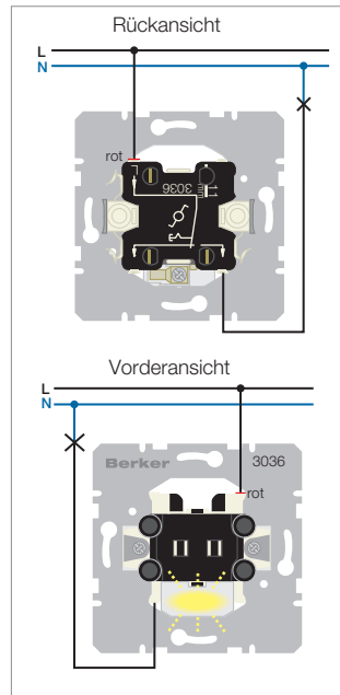
Ausschaltung Beleuchtet mit Wechselschalter (Glimmaggregat leuchtet bei "Aus")
