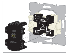
Serien-LED-Aggregat von hinten aufrasten.
