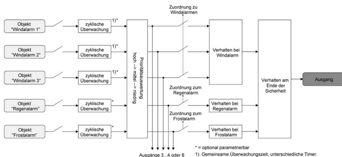
Bild 18: Funktionsschaltbild der kanalorientierten Sicherheitsfunktionen
