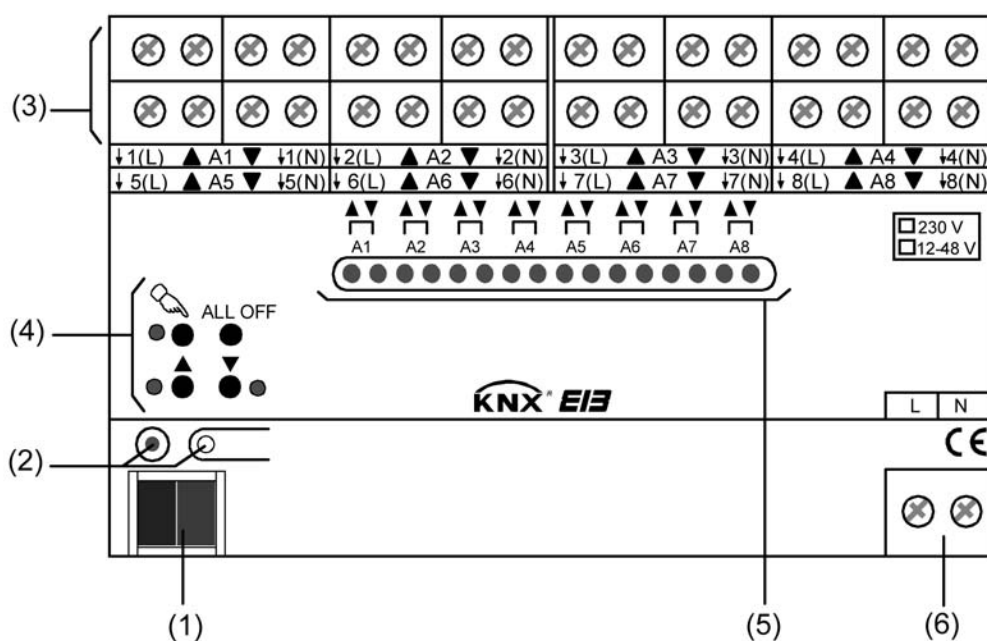
Bild 2: Geräteaufbau des Jalousieaktors 4/8fach REG
