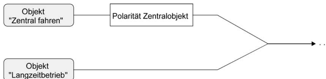
Bild 9: Funktionsschaltbild "Zentral fahren"
