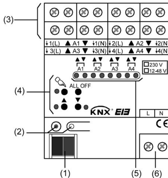
Bild 1: Geräteaufbau des Jalousieaktors 2/4fach REG
