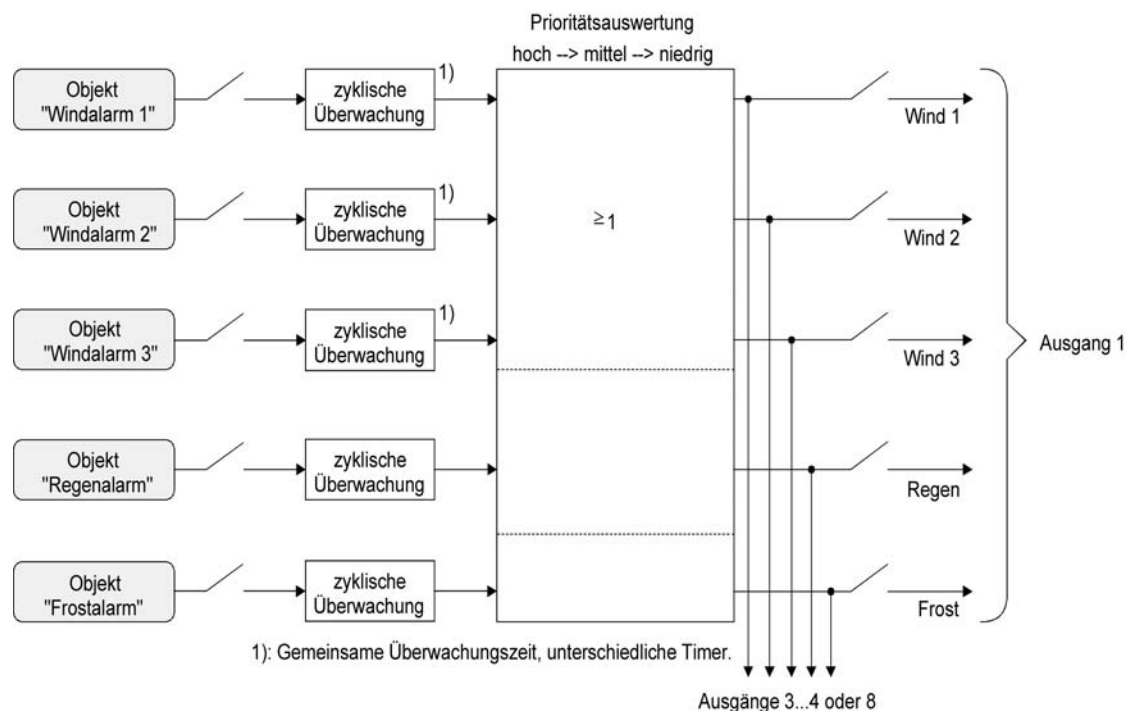
Bild 10: Funktionsschaltbild der Sicherheitsfunktionen
