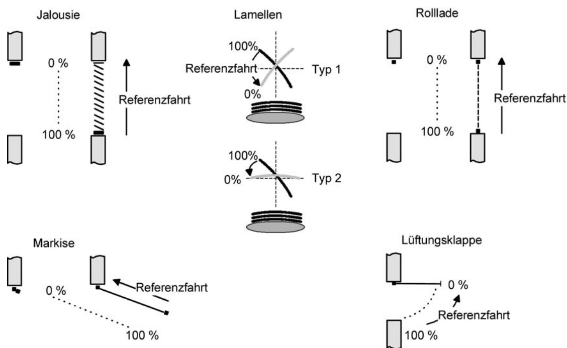
Bild 17: Referenzfahrt
