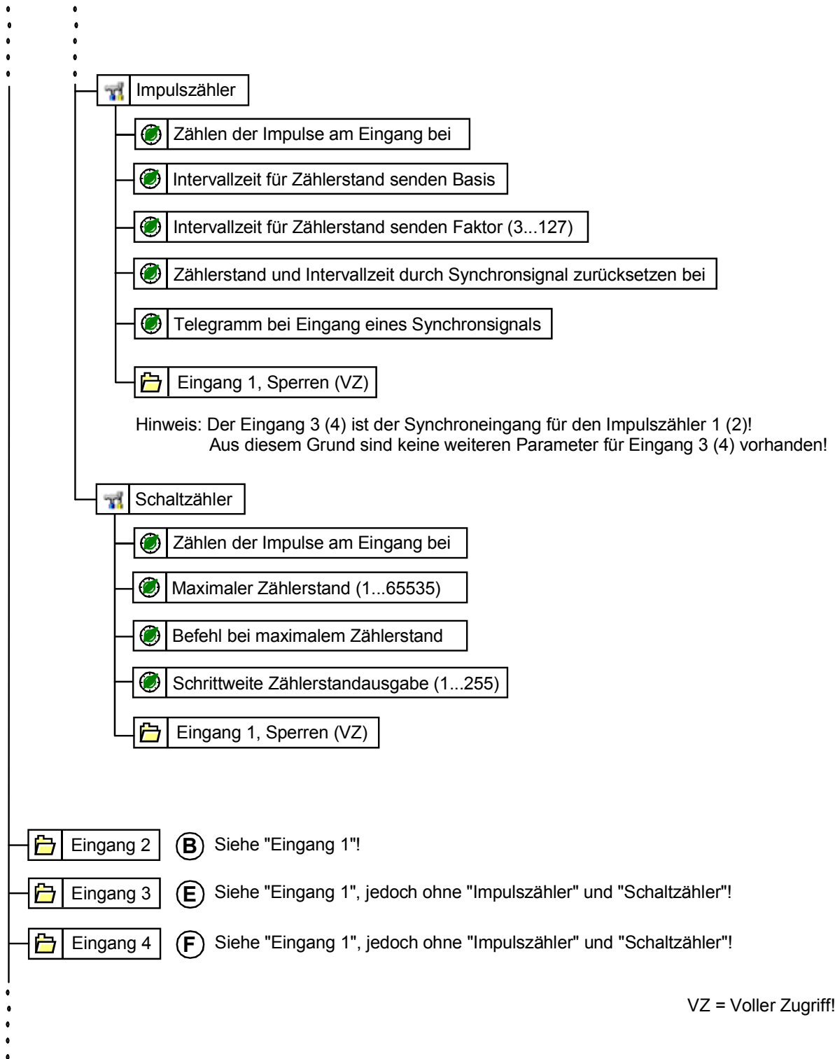
Parameterbild (Bild 6 von 8)
