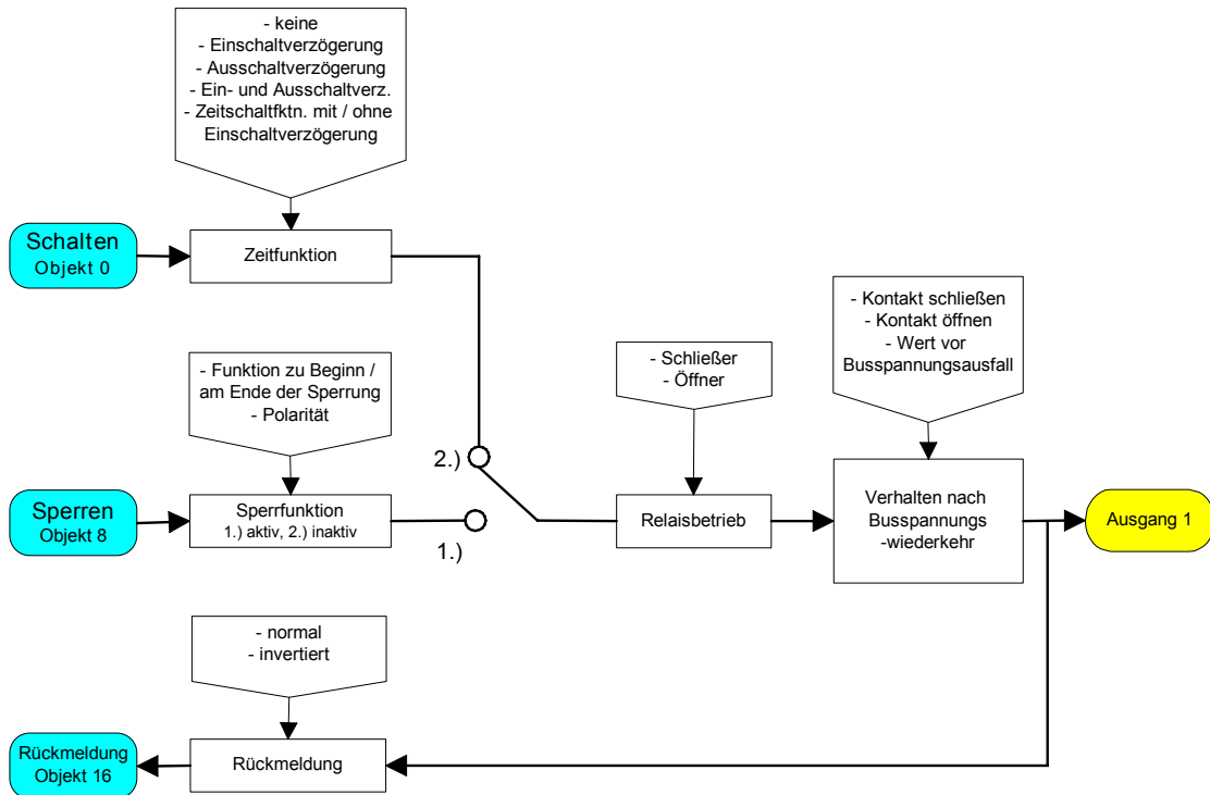
Funktionsschaltbild (für Schaltausgänge / z. B. Ausgang 1 mit der Zusatzfunktion "Sperrobjekt")
