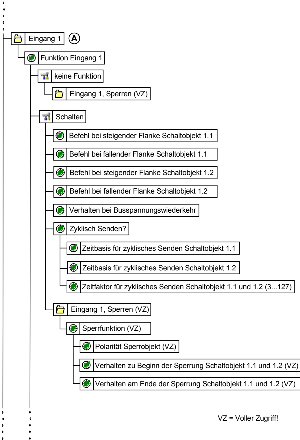
Parameterbild (Bild 2 von 8)
