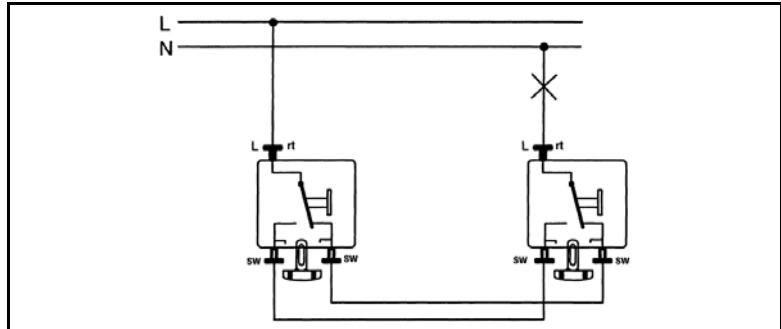
Anschlussbeispiel 606 NAW 606 NAW
