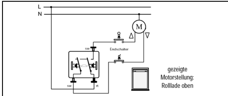
Anschlussbeispiel 609 VA
