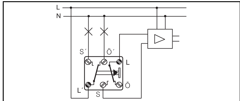
Anschlussbeispiel 639 W
