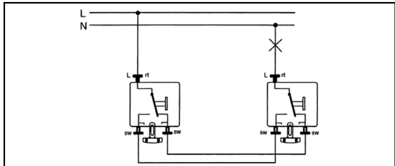
Anschlussbeispiel 806 NAW
