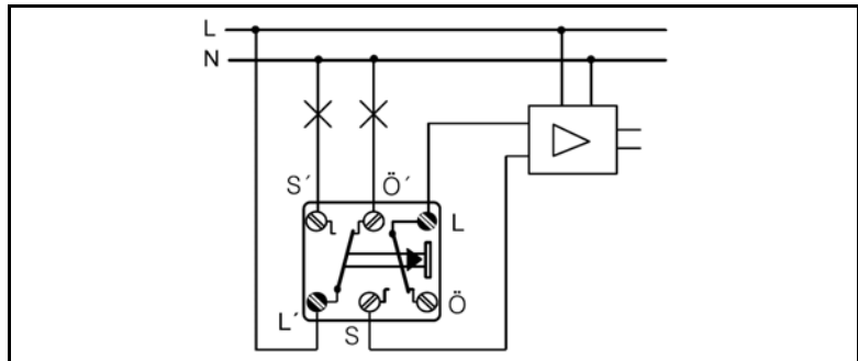
Anschlussbeispiel 833-2 W
