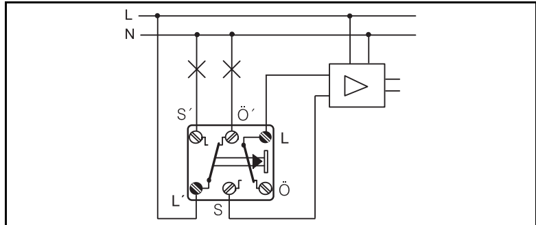
Anschlussbeispiel 839 W
