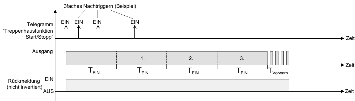
Bild 14: Zeitverlängerung der Treppenhausfunktion
