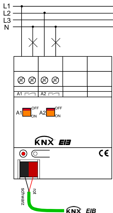
Bild 1: Elektrischer Anschluss
