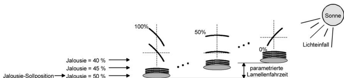
Bild 15: Beispiel für Lamellenpositionierung mit Auswirkung auf die Jalousieposition (Beispielhaft für Lamellentyp 1. Typ 2 sinngemäß gleich.)
