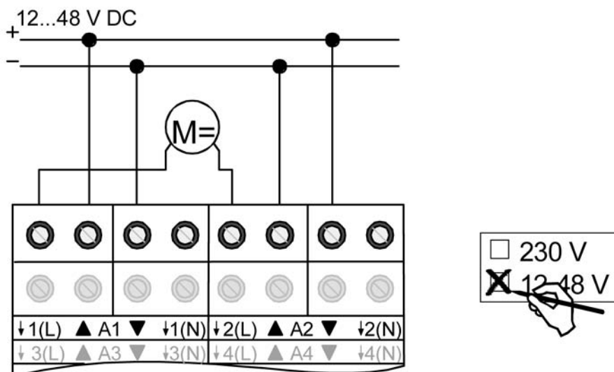
Bild 6: Elektrischer Anschluss für 12 ... 48 V-Antriebsmotoren
