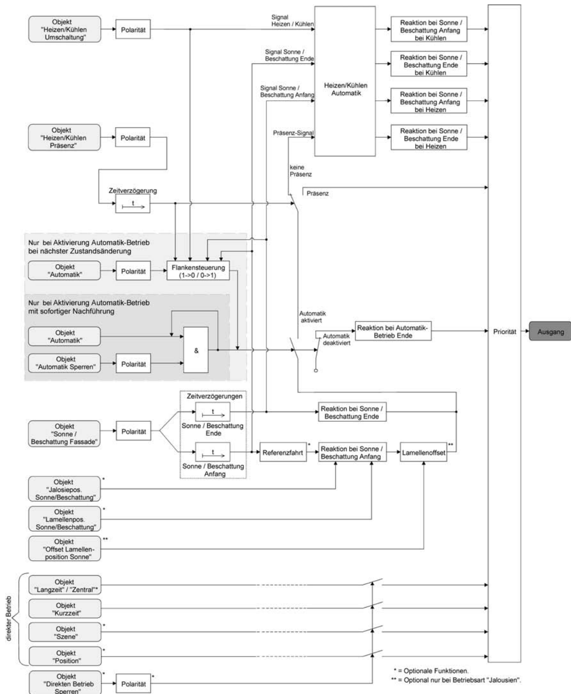
Bild 26: Funktionsschaltbild der Heizen/Kühlen-Automatik
