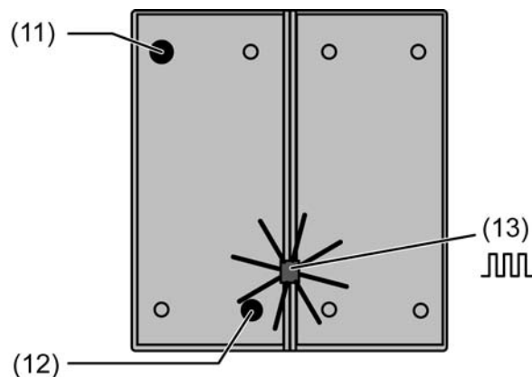
Bild 3: Tasten zur Aktivierung des Programmiermodus
