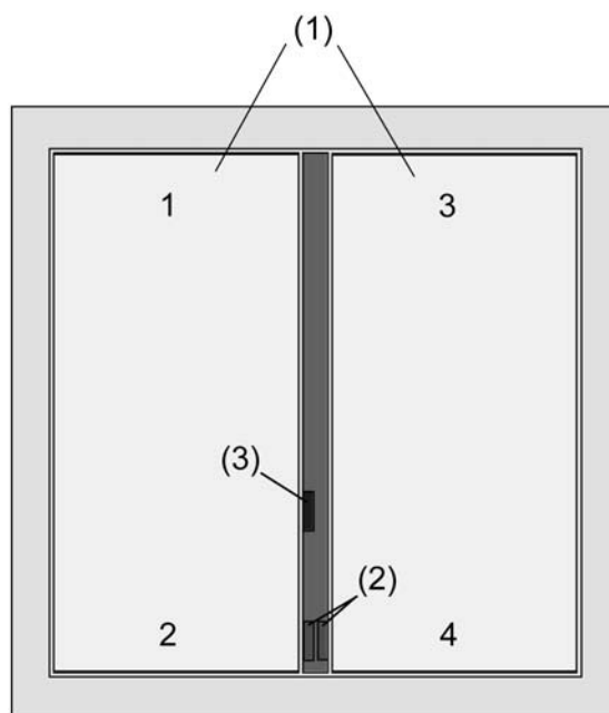
Bild 1: Geräteanordnung Tastsensor 2fach Standard TSM
